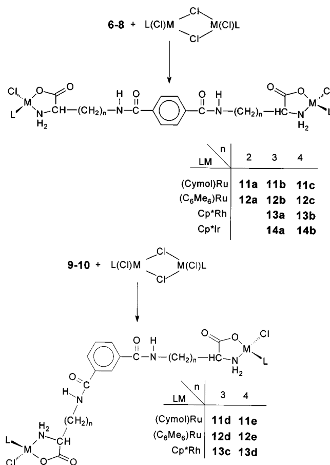
Schema 3 Synthese der ligandverbrückten Halbsandwich-Komplexe 11–14
