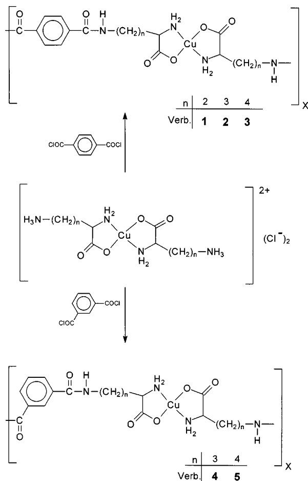
Schema 1 Bildung der polymeren Bis( \alpha -aminocarboxylat)-Kupfer-Komplexe 1–5
