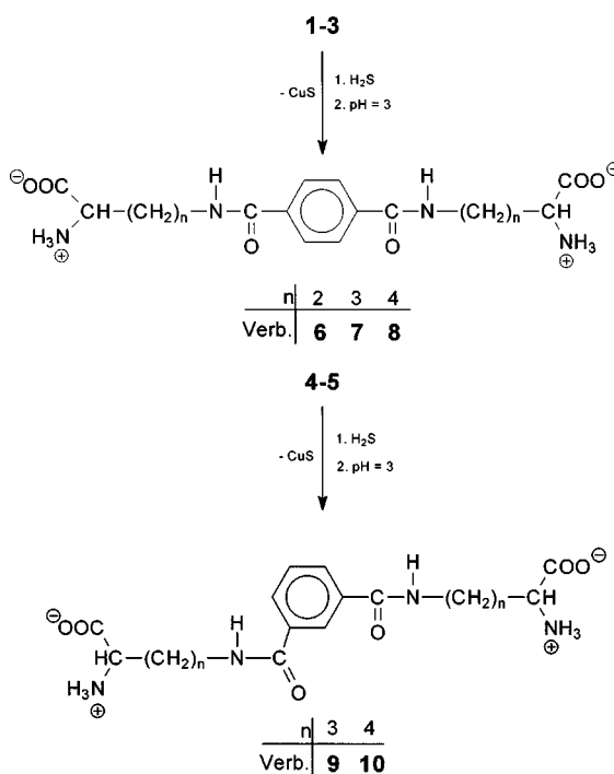
Schema 2 Synthese der Phthaloylverbrückten Lysin- und Ornithin-Liganden 6–10
